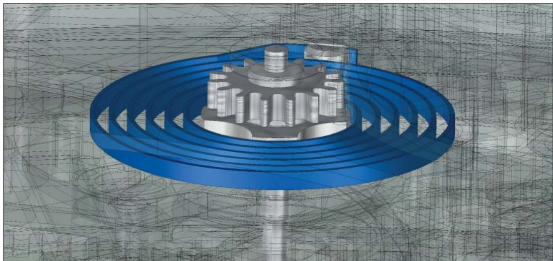
Die Funktionsüberprüfung erfolgt im Umfeld des restlichen Uhrwerks. So lassen sich Kollisionen sicher vermeiden.
